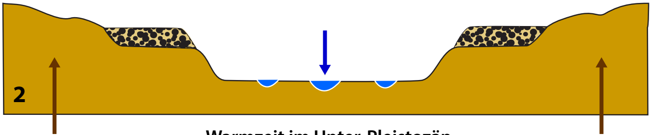
Warmzeit im Unter-Pleistozän vor mehr als 700 000 Jahren
