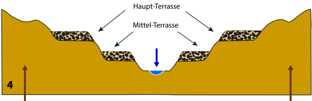
Warmzeit im Holozän vor 11 700 Jahren bis heute
