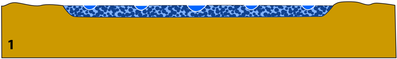
Eiszeit im Unter-Pleistozän vor mehr als 1 Mio Jahren
