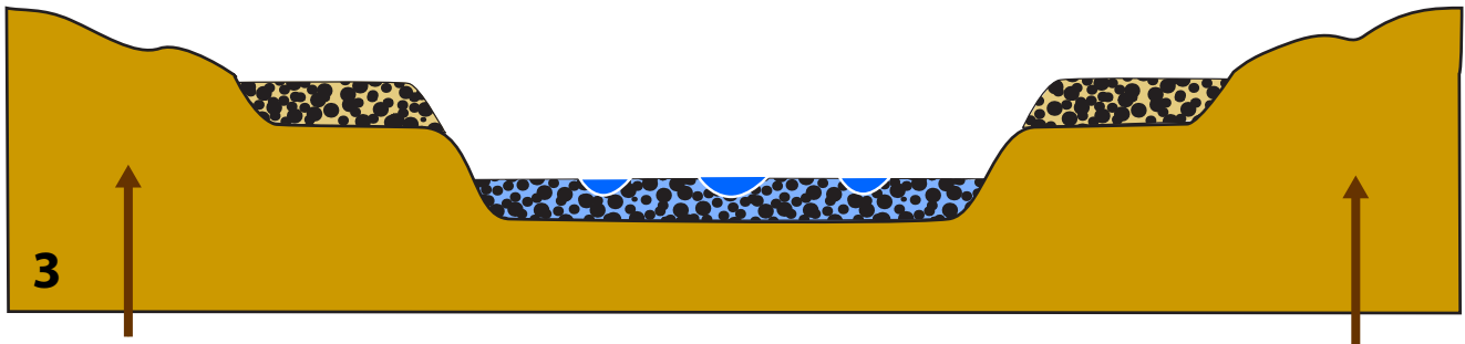
Saale-Eiszeit vor 250 000 bis 128 000 Jahren
